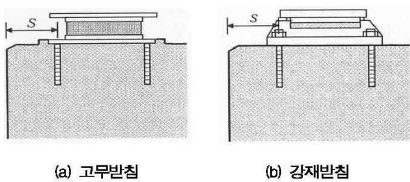
【그림 27.3.2】 도로교설계기준 연단거리 산출방법
