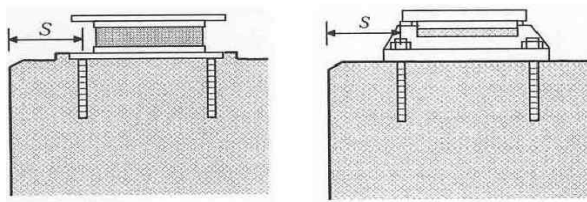
(a) 고무받침
