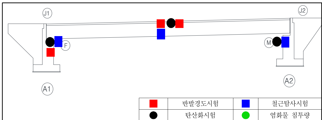
【그림 27.4.2】 영천방향 콘크리트 내구성조사 위치도
